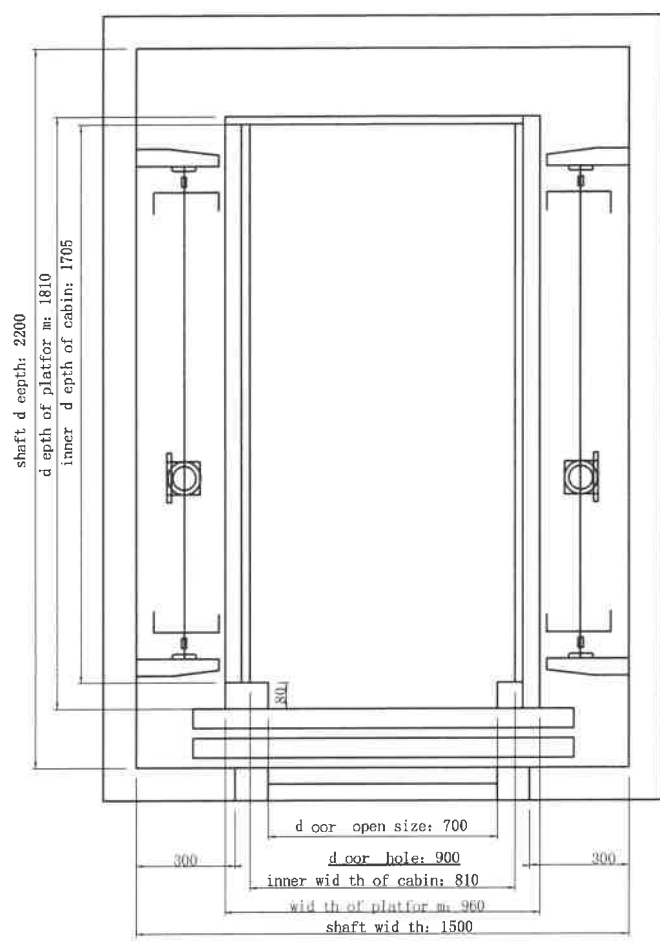
井道平面图
