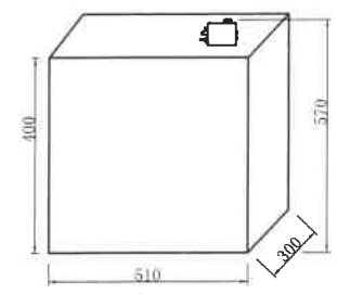
泵站示意图
